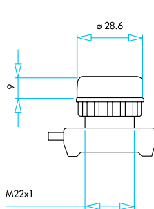
Düz, Yaylı Flush, Spring Return
