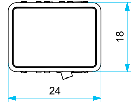
Dikdörtgen Buton Rectangle Button
