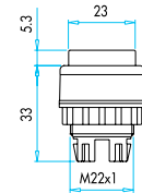
Çıkık Kafalı Extended, Spring Return
