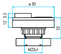
Çiftli Çıkık Kafalı Double Extended, Spring Return
